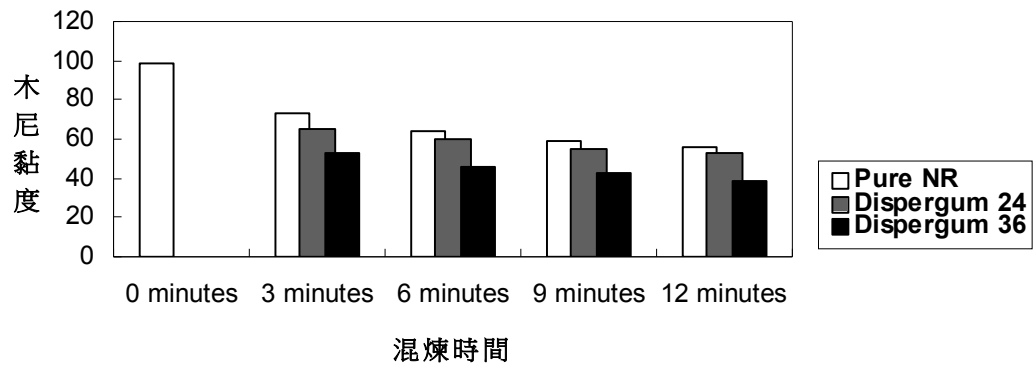
天然橡膠在 80°C 之素煉
